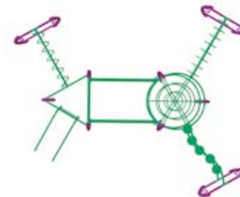
DISCOVERY EXTRE-5 Capacidad: 36 usuarios Medidas: L: 7.00 m / An: 5.70 m / Al: 2.80 m
