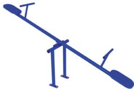
SUBE Y BAJA SENCILLO SYB01 Capacidad: 2 usuarios Medidas: L: 2.30 m / An: 0.50 m / Al: 1.20 m
