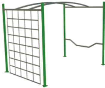
ESCALADOR Y PASAMANOS JIMCR-05 Capacidad: 7 usuarios L: 3.20 m / An: 2.10 m / Al: 2.40 m
