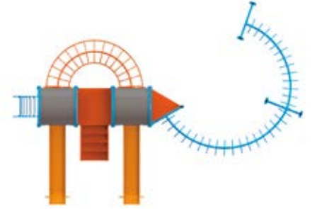
ORBIT TM10B Capacidad: 35 usuarios Medidas: L: 8.10 m / An: 5.60 m / Al: 3.90 m Área de seguridad: L: 10.10 m / An: 8.10 m
