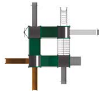
MULTICUPULA TM07B Capacidad: 40 usuarios Medidas: L: 8.30 m / An: 7.70 m / Al: 4.20 m Área de seguridad: L: 11.30 m / An: 10.70 m
