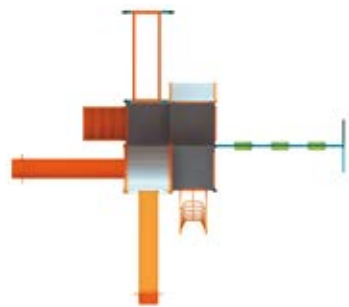
MULTITORRE TM02B Capacidad: 33 usuarios Medidas: L: 7.80 m / An: 6.80 m / Al: 4.20 m Área de seguridad: L: 10.80 m / An: 9.80 m
