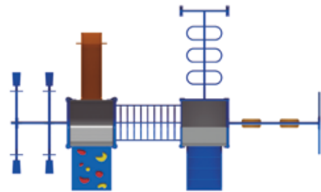
CANDY TM01B Capacidad: 25 usuarios Medidas: L: 6.90 m / An: 4.00 m / Al: 3.50 m Área de seguridad: L: 8.90 m / An: 6.00 m
