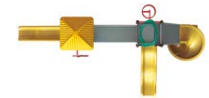
PACHAL NO. 6 Accesorios plásticos TM83P Capacidad: 22 usuarios Medidas: L: 8.30 m / An: 4.00 m / Al: 3.70 m Área de seguridad: L: 10.30 m / An: 6.00 m
