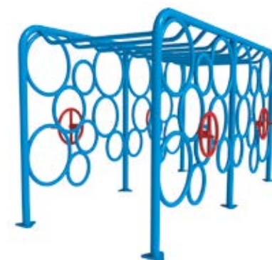
TUNEL PASAMANOS INC-04 Capacidad: 6 usuarios Medidas: L: 2.90 m / An: 1.60 m / Al: 1.60 m Área de seguridad: L: 5.90 m / An: 4.60 m
