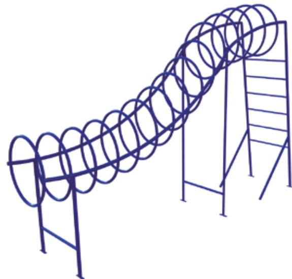
GUSANO TPD06 Capacidad: 6 usuarios Medidas: L: 3.40 m / An: 0.65 m / Al: 2.00 m Área de seguridad: L: 5.40 m / An: 2.65 m
