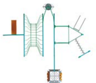
VOLCANO Accesorios plásticos EXTRE-6 Capacidad: 40 usuarios Medidas: L: 9.60 m / An: 8.70 m / Al: 2.80 m
