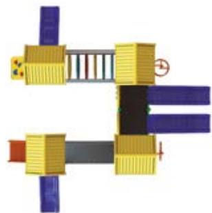
PACHAL NO. 8 Accesorios plásticos TM85P Capacidad: 44 usuarios Medidas: L: 7.60 m / An: 7.40 m / Al: 3.50 m Área de seguridad: L: 9.60 m / An: 9.40 m
