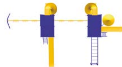
TORRE MULTIJUEGO 06 Accesorios en fibra en vidrio TM-006 Capacidad: 38 usuarios Medidas: L: 10.50 m / An: 5.80 m / Al: 4.30 m Área de seguridad: L: 13.50 m / An: 8.80 m
