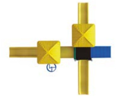
PACHAL NO. 3 Accesorios plásticos TM80P Capacidad: 24 usuarios Medidas: L: 6.70 m / An: 6.10 m / Al: 3.50 m Área de seguridad: L: 8.70 m / An: 8.10 m
