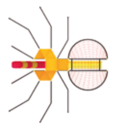
ARAÑA Accesorios plásticos TMA01 Capacidad: 60 usuarios Medidas: L: 9.00 m / An: 10.00 m / Al: 3.00 m Área de seguridad: L: 12.00 m / An: 13.00 m
