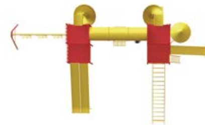
TORRE MULTIJUEGO 05 TM-005 Accesorios en fibra en vidrio Capacidad: 40 usuarios Medidas: L: 10.50 m / An: 6.20 m / Al: 4.30 m Área de seguridad: L: 13.50 m / An: 9.20 m
