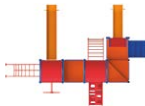
VIENA TM06B Capacidad: 34 usuarios Medidas: L: 6.10 m / An: 4.70 m / Al: 4.20 m Área de seguridad: L: 8.10 m / An: 7.20 m
