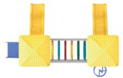
PACHAL NO. 1 Accesorios plásticos TM78P Capacidad: 18 usuarios Medidas: L: 3.50 m / An: 5.10 m / Al: 3.20 m Área de seguridad: L: 5.50 m / An: 7.10 m
