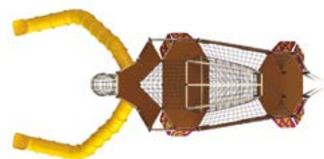
MAMUT Accesorios plásticos TMA09 Capacidad: 100 usuarios Medidas: L: 15.50 m / An: 7.50 m / Al: 7.50 m Área de seguridad: L: 20.00 m / An: 13.00 m
