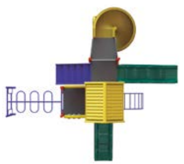
PACHAL NO. 2 TM79P Accesorios Plásticos Capacidad: 26 usuarios Medidas: L: 6.30 m / An: 5.50 m / Al: 3.70 m Área de seguridad: L: 8.30 m / An: 7.60 m
