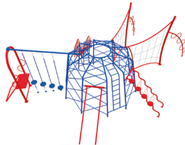
SKY EXTRE-2 Capacidad: 45 usuarios Medidas: L: 9.20 m / An: 6.20 m / Al: 2.80 m
