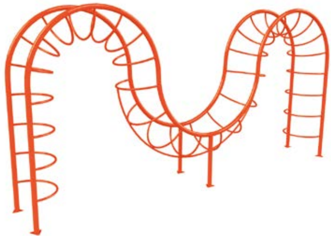
TREPADERO DE JOROBAS TPD01 Capacidad: 7 usuarios Medidas: L: 4.00 m / An: 0.60 m / Al: 1.95 m Área de seguridad: L: 6.00 m / An: 2.60 m
