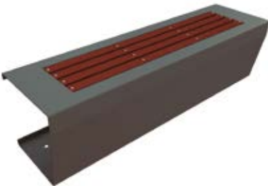
SALVORA BASAE-150 Capacidad: 3 usuarios L: 1.50 m / An: 0.41 m / Al: 0.41 m
