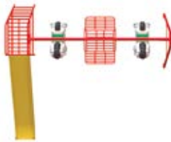
JUEGO DE CONJUNTO 03 JCO03 Capacidad: 6 usuarios Medidas: L: 3.00 m / An: 1.40 m / Al: 2.00 m Área de seguridad: L: 5.00 m / An: 4.20 m
