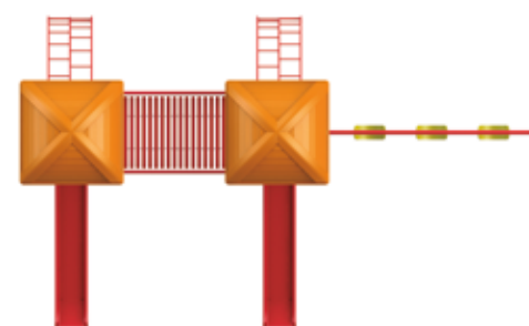
MENA TM011 Capacidad: 21 usuarios Medidas: L: 7.10 m / An: 4.20 m / Al: 3.70 m Área de seguridad: L: 9.10 m / An: 6.70 m
