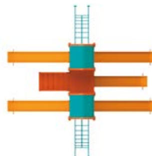
UP-DOWN TM09B Capacidad: 28 usuarios Medidas: L: 5.20 m / An: 5.00 m / Al: 3.80 m Área de seguridad: L: 8.20 m / An: 7.00 m
